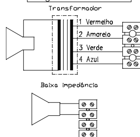
Transformador 100 Volt linha Derivação primário
